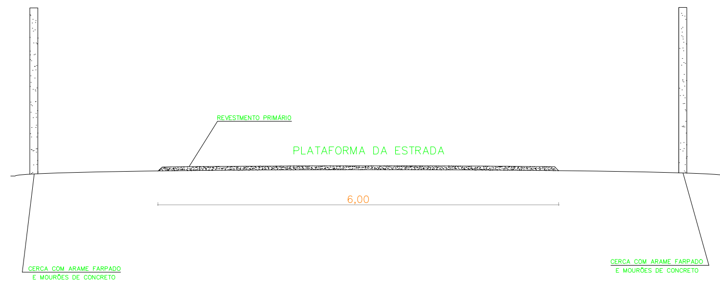
SEÇÃO TRANSVERSAL – IMPLANTAÇÃO DO REVESTIMENTO PRIMÁRIO S/ ESCALA
