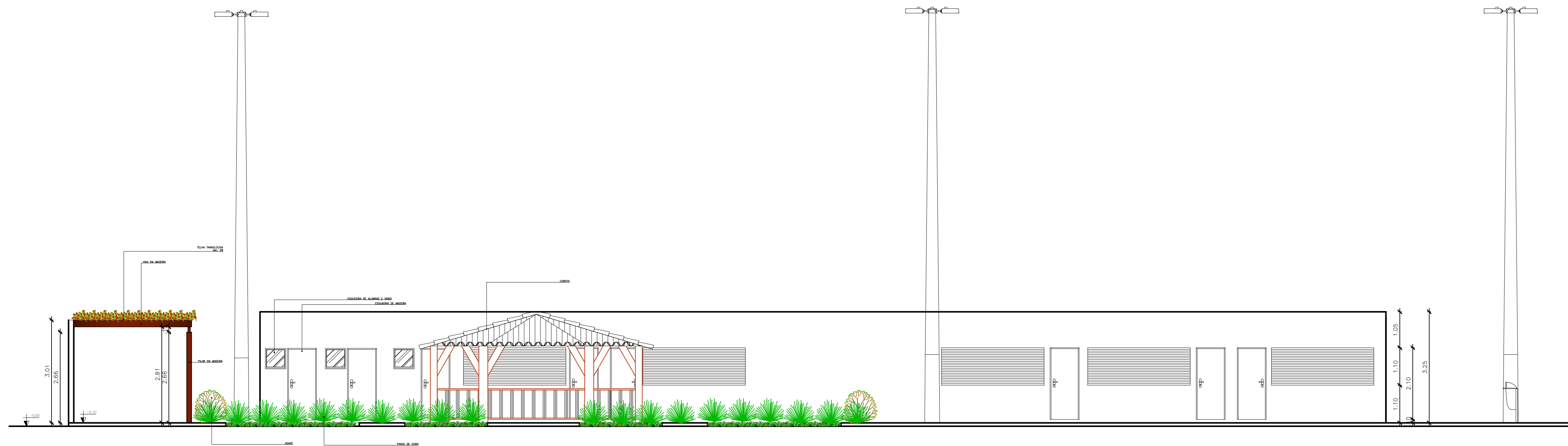
CORTE BB ESC.: 1/175
