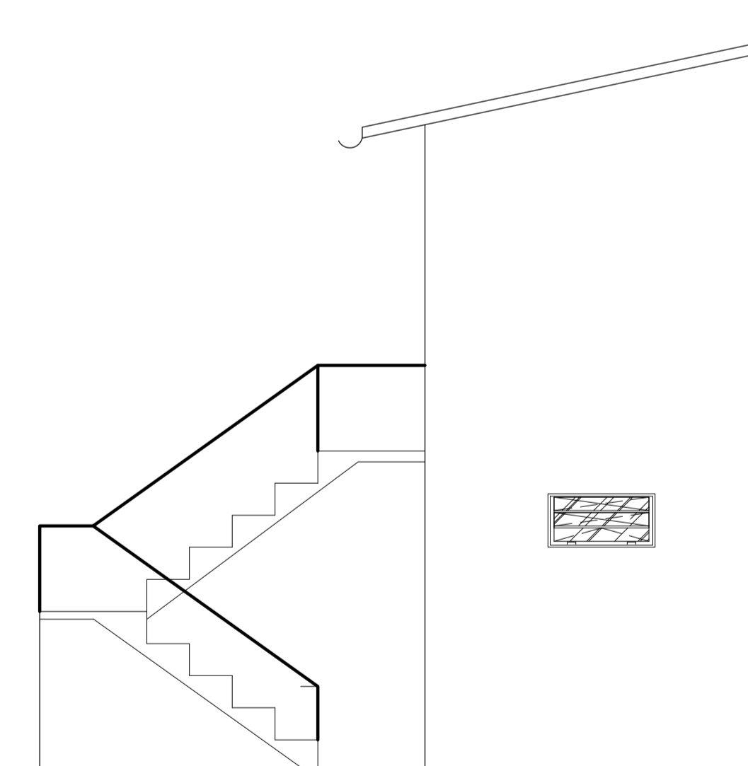
FACHADA LATERAL ESC.: 1/50
