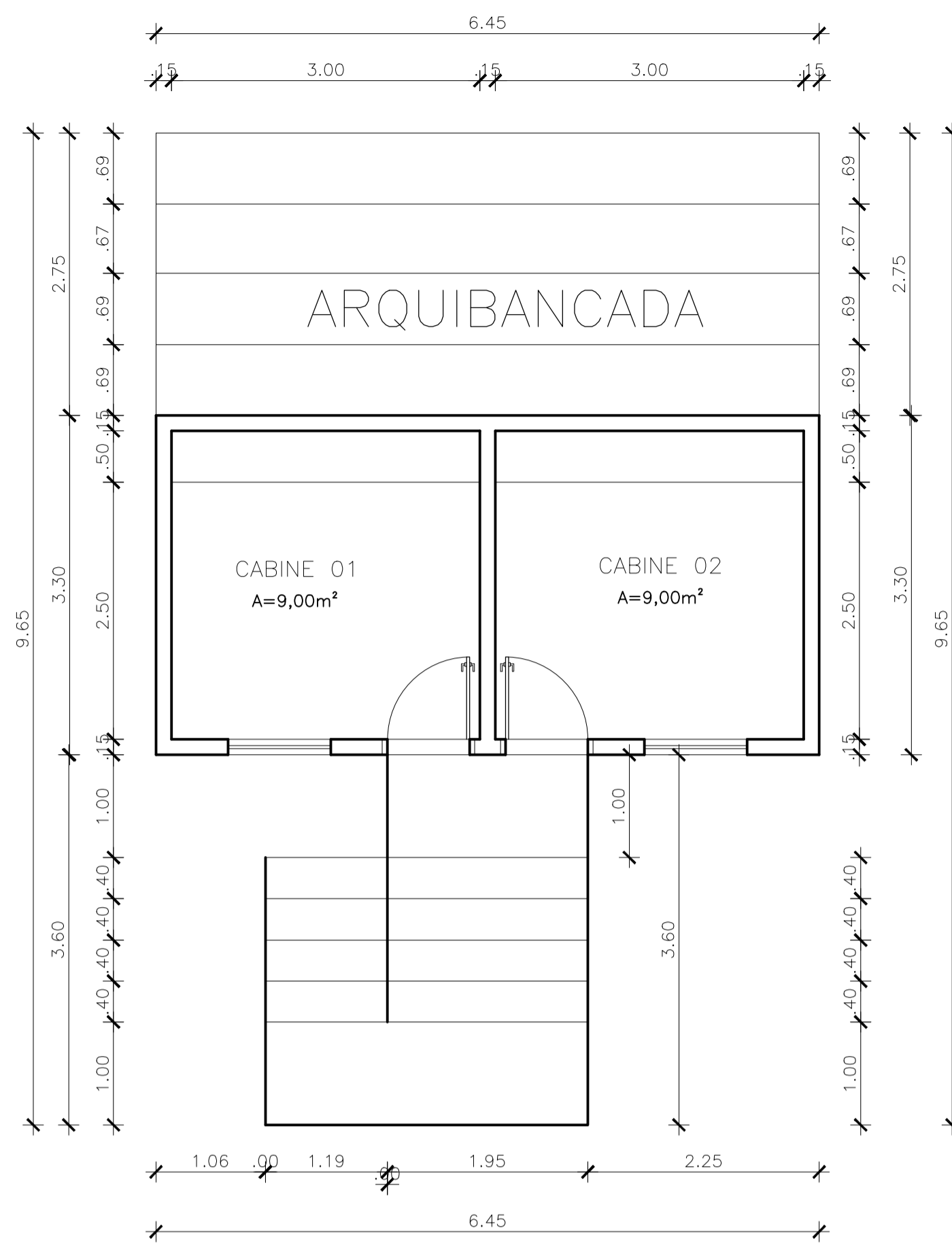
PLANTA BAIXA – CABINES – PISO SUPERIOR ESC.: 1/50
