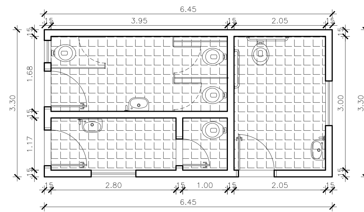
PLANTA BAIXA – CABINES – PISO INFERIOR ESC.: 1/50
