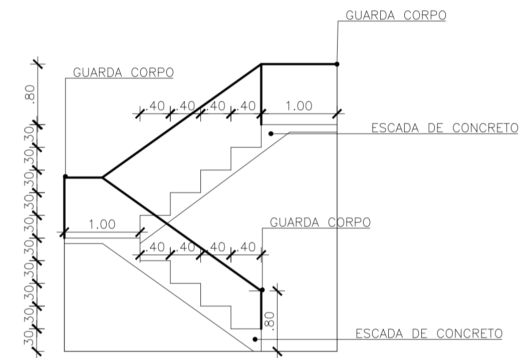
DETALHAMENTO DA ESCADA ESC.: 1/50
