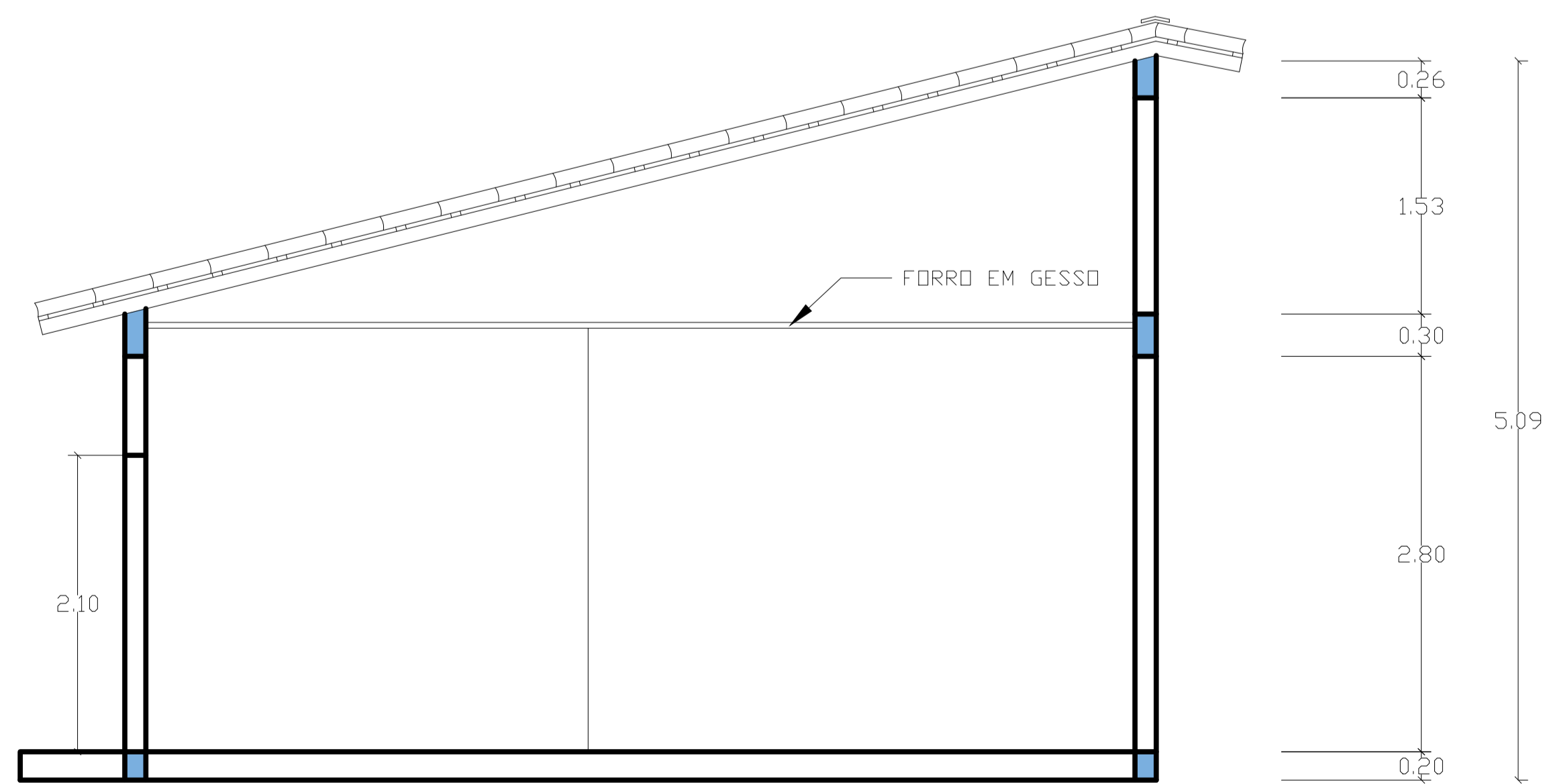
CORTE C-C'
