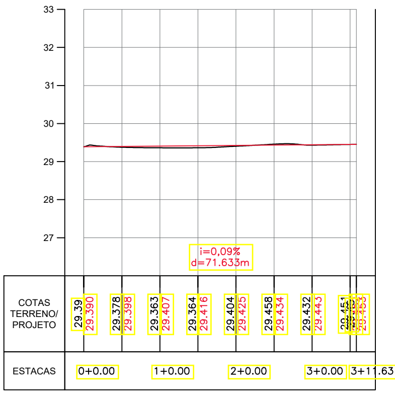
D/2 PERFIL LONGITUDINAL Escala: 1/1.000
