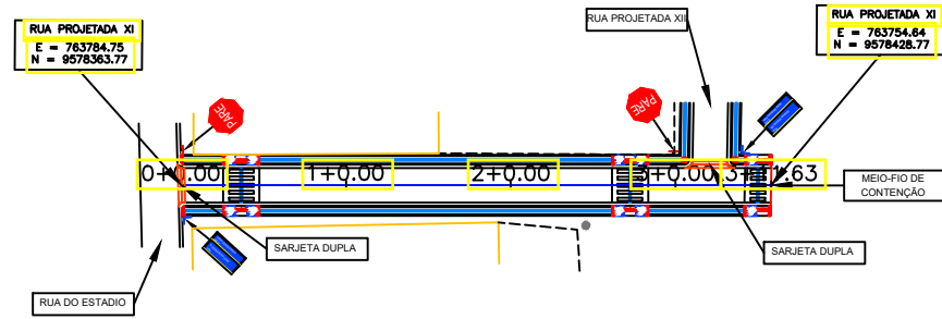
D/1 TRAÇADO HORIZONTAL Escala: 1/1.000
