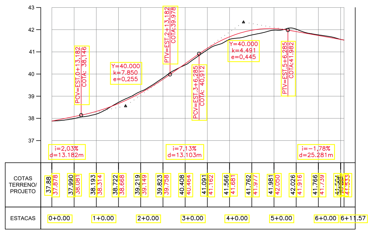
D/2 PERFIL LONGITUDINAL Escala: 1/1.000
