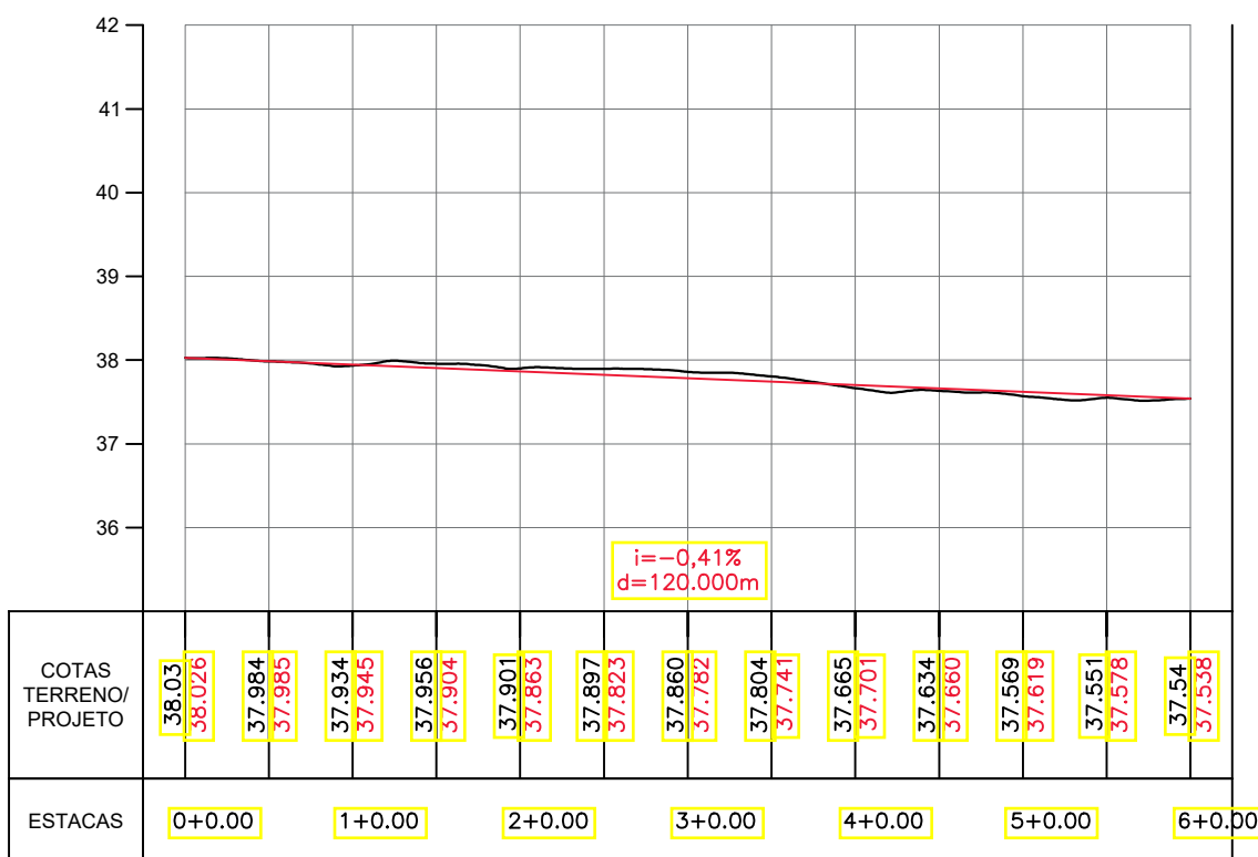
D/2 PERFIL LONGITUDINAL Escala: 1/1.000
