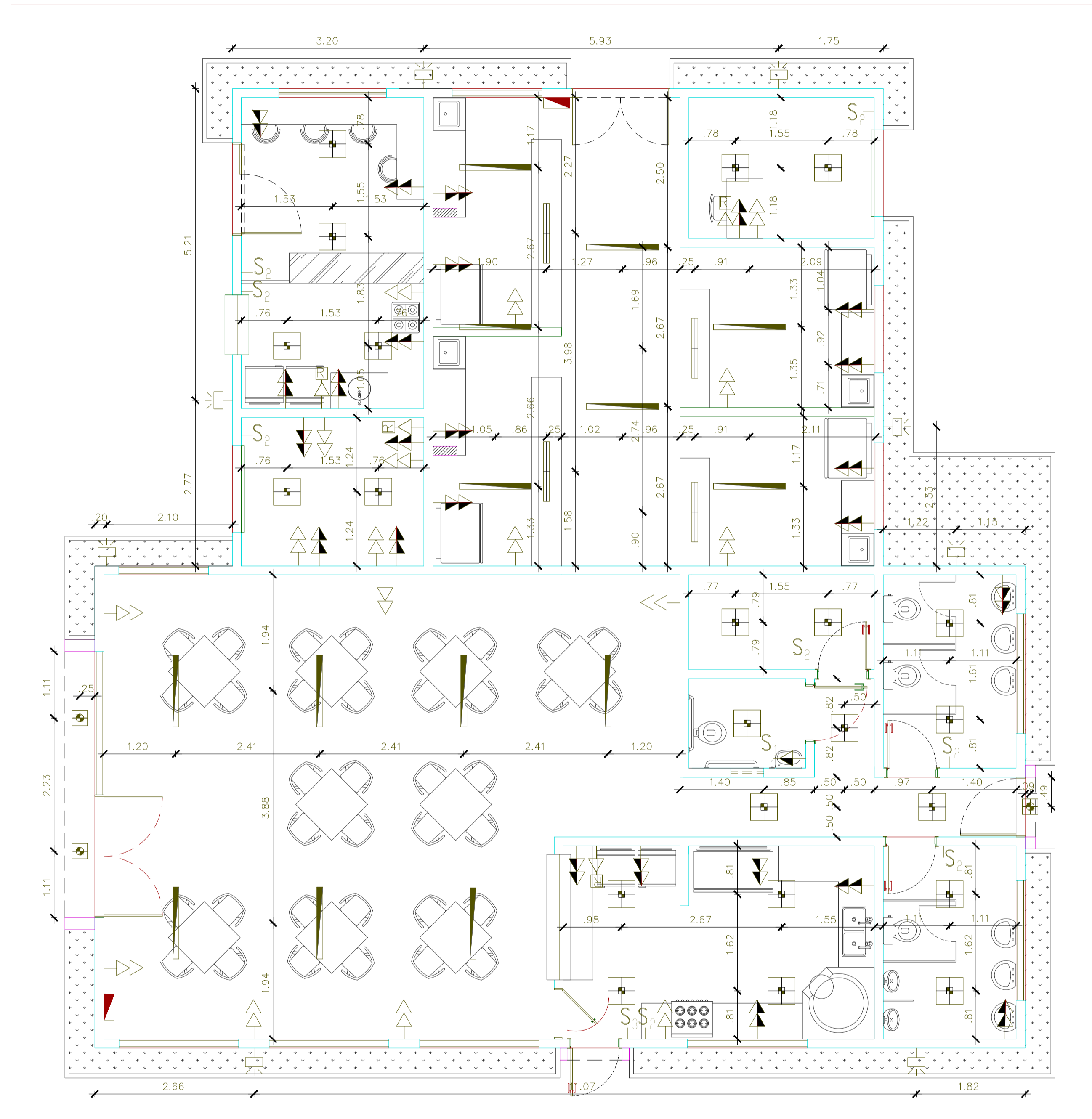
PLANTA DE PONTOS ELÉTRICOS/LUMINÁRIAS ESC.: 1/75
