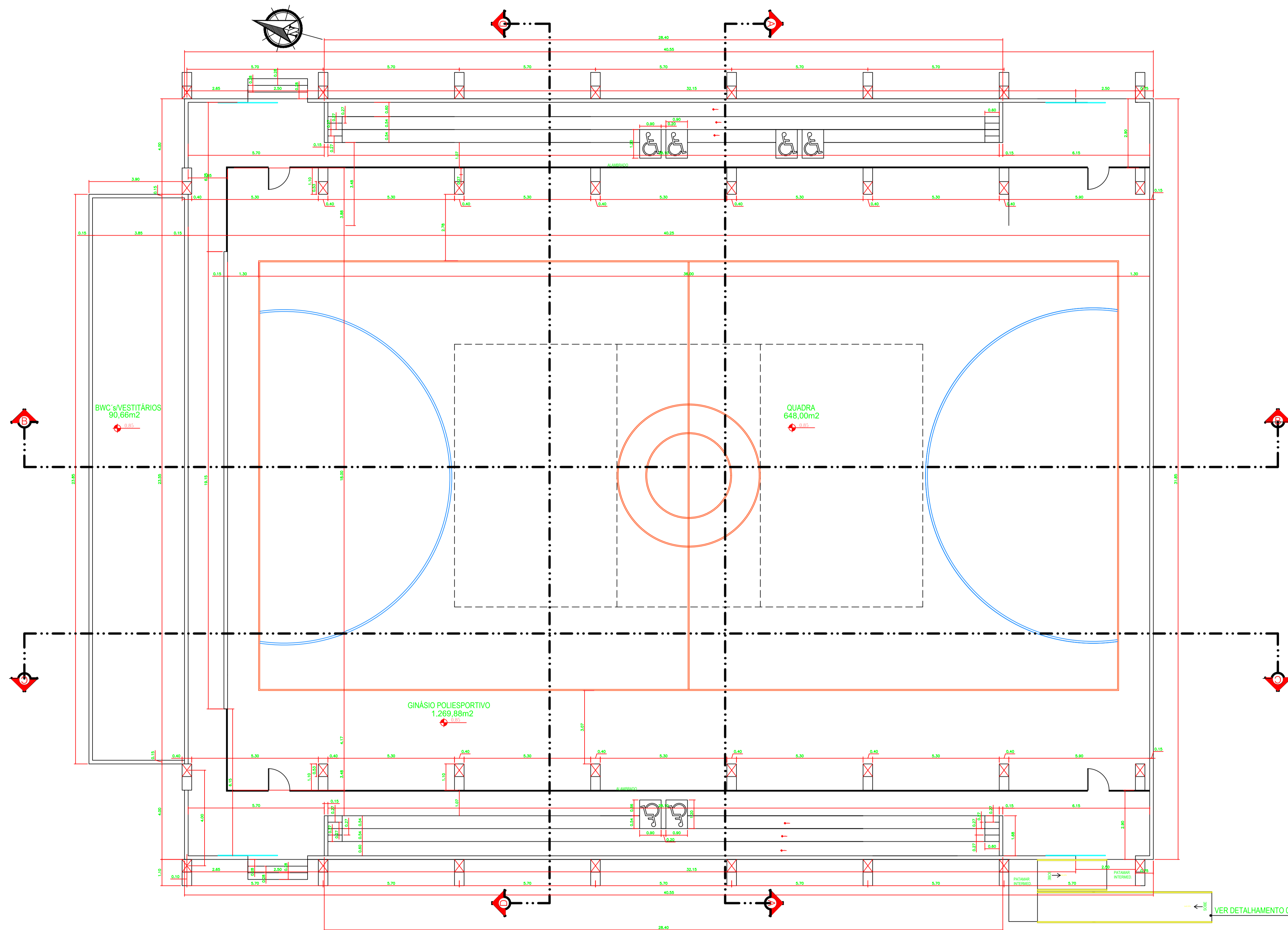
PLANTA BAIXA SITUAÇÃO PRETENDIDA Esc. 1:100
